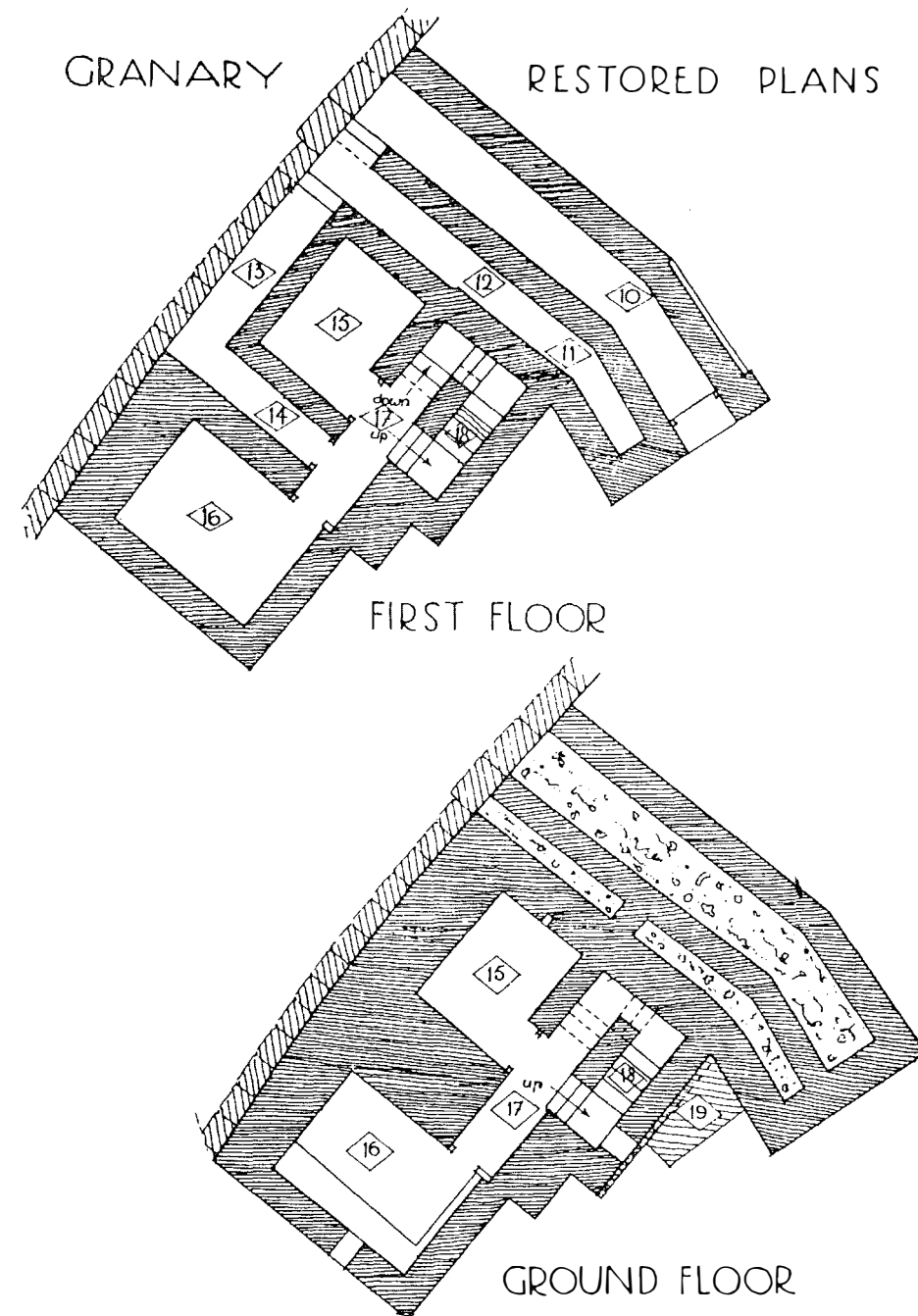
Εικ. 4. Μυκίναι, Σιταποθήκη, κάτοψις ισογείου (υπογείου) και πρώτου ορόφου (Wace 1949, Fig. 3).
