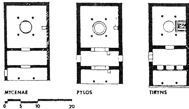
Εικ. 5. Κατόψεις μεγάλων Μυκηνών, Πύλου, Τίρυνθος (Μυλωνάς 1966, Fig. 16).
