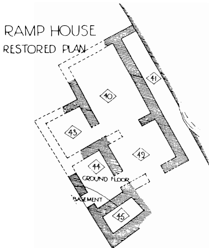
Εικ. 9. Μυκήναι, Οικία Αναβάθρας, κάτοψις (Wace 1949, Fig. 3).
