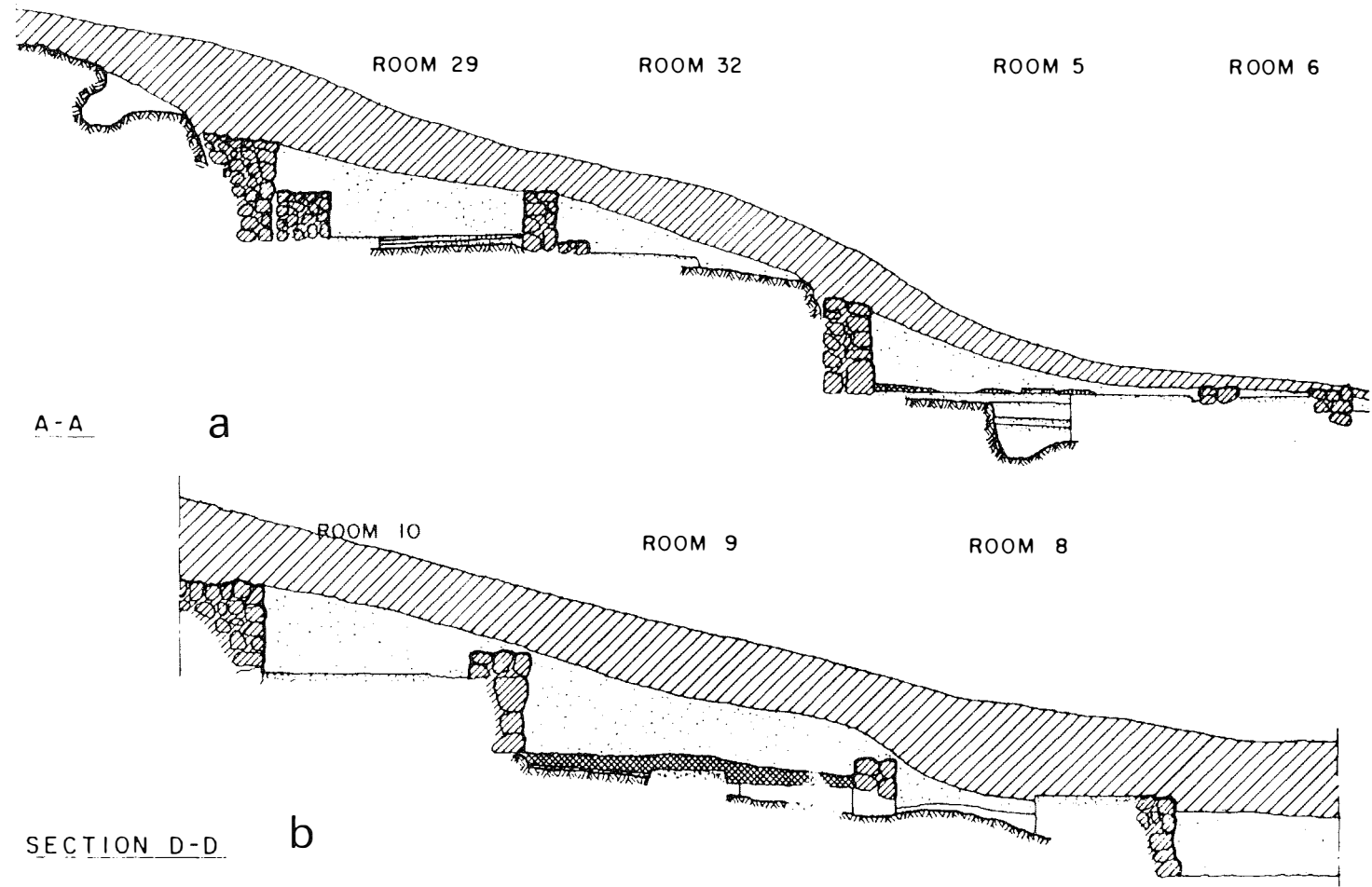
17. Μυκήναι, Οικίες λόφου Παναγίας (Mylonas-Shear 1987) α) Τομή Α-Α (Οικία ΙΙΙ, Οικία Ι). β) Τομή Δ-Δ (Οικία ΙΙ).
