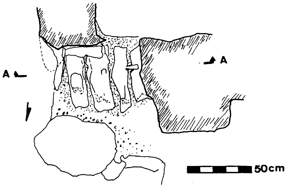
Εικ. 20. Μυκίναι, εστία Δυτικής Οικίας, κάτοψις, τομή (Βερδελής 1959, Εικ. 5).
