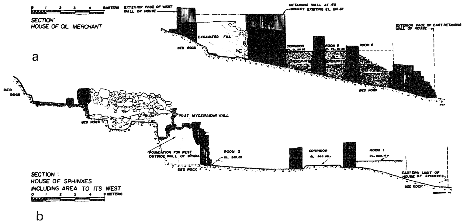
Εικ. 16. Μυκήναι α) Οικία Λαδεμπόρου, τομή Δ-Α (Chadwick 1962, Plan IV). β) Μυκήναι, Οικία Σφιγγών, τομή Δ-Α (Chadwick 1962, Plan IV).
